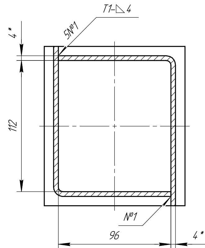
Б-Б
