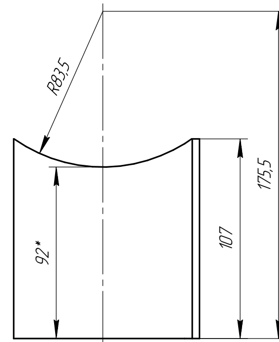
Дет. поз. 2
