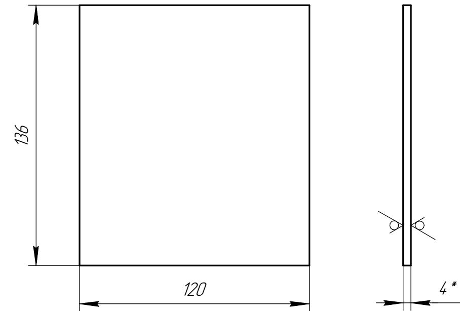
Дет. поз. 1
